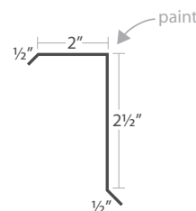
Mini Gable
